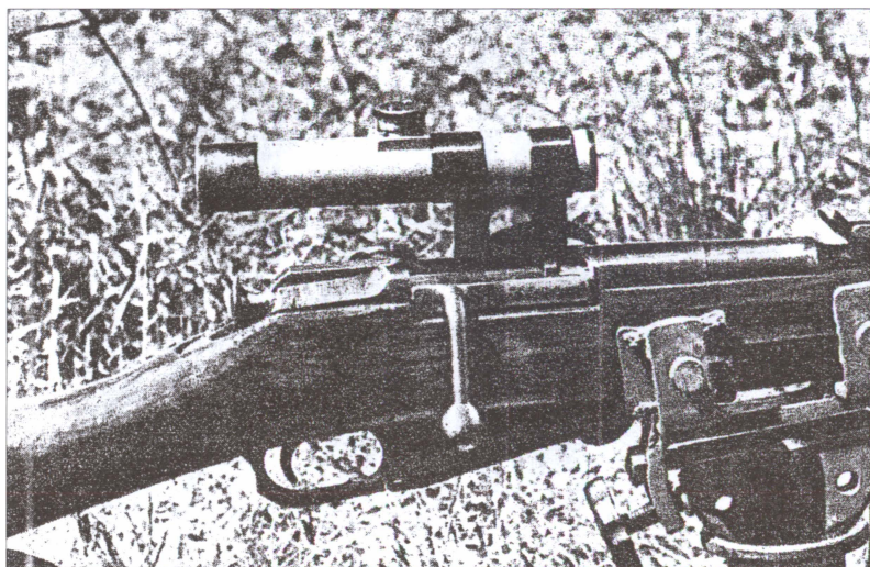
Оптический прицел Емельянова («ПЕ»), установленный на винтовке СВТ-38
