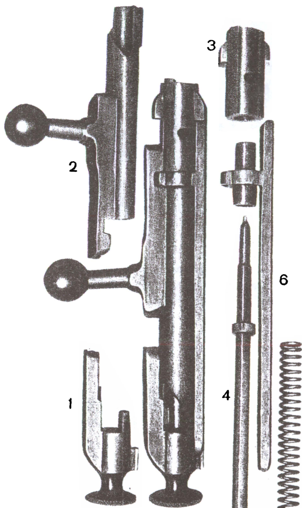
Продольно-скользящий затвор винтовки Мосина и его части: 1 — курок; 2 — стебель затвора с рукояткой; 3 — боевая личинка; 4 — к курку привинчивается ударник с бойком; 5 — на ударник надевается боевая пружина; 6 — эта планка соединяет части затвора; она и называется соединительной
