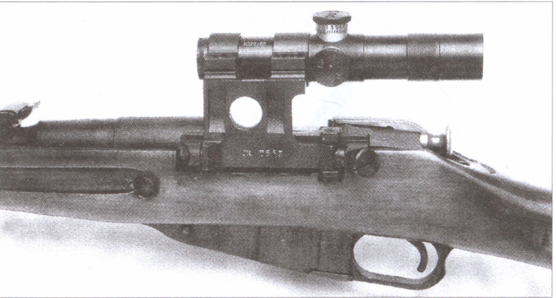
Прицел «ПУ» на винтовке Мосина. Вид слева
