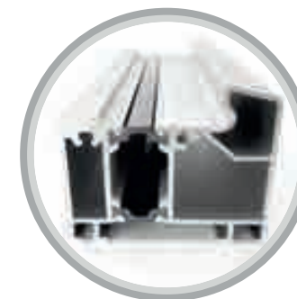
АЛЮМІНІЄВИЙ ПОРІГ 50 ММ З ТЕРМОРОЗРИВОМ
