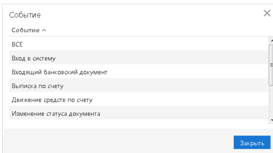
Рис. 8. Диалог "Событие"
