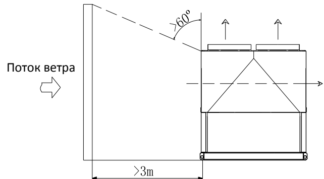
установка ветрозащитных ограждений
