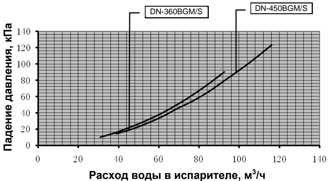
Графики падения давления воды в испарителе
