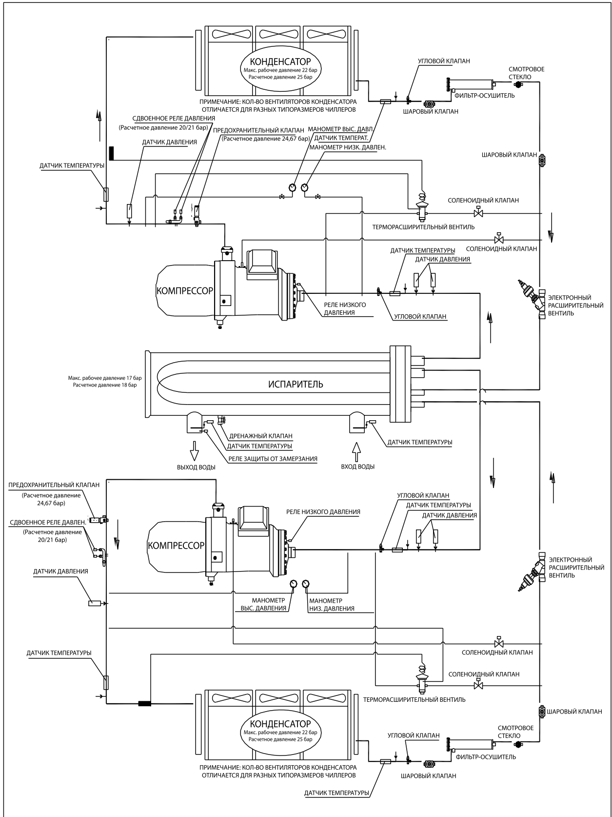
ПРИЛОЖЕНИЕ - ПРИНЦИПАЛЬНАЯ ТЕХНОЛОГИЧЕСКАЯ СХЕМА ДВУХКОМПРЕССОРНЫХ ЧИЛЛЕРОВ
