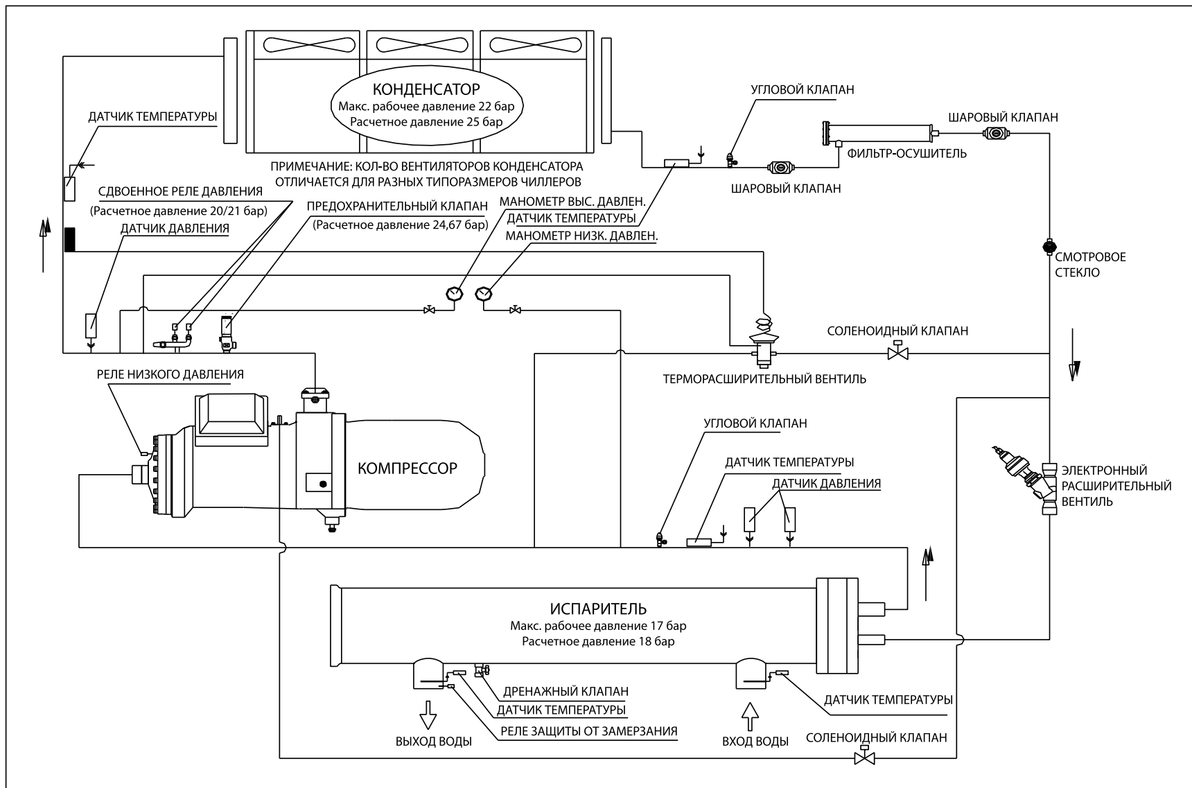
ПРИЛОЖЕНИЕ - ПРИНЦИПАЛЬНАЯ ТЕХНОЛОГИЧЕСКАЯ СХЕМА ОДНОКОМПРЕССОРНЫХ ЧИЛЛЕРОВ
