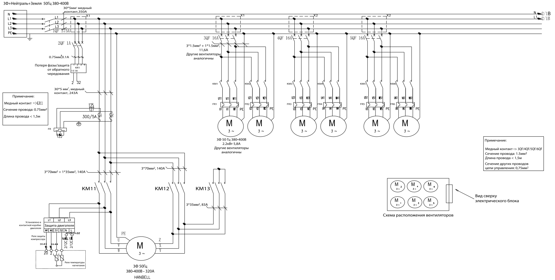
Электросхема для DN360BGM/S
