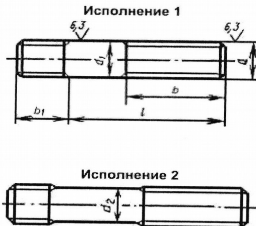
Чертеж. Конструкция и размеры шпилек
