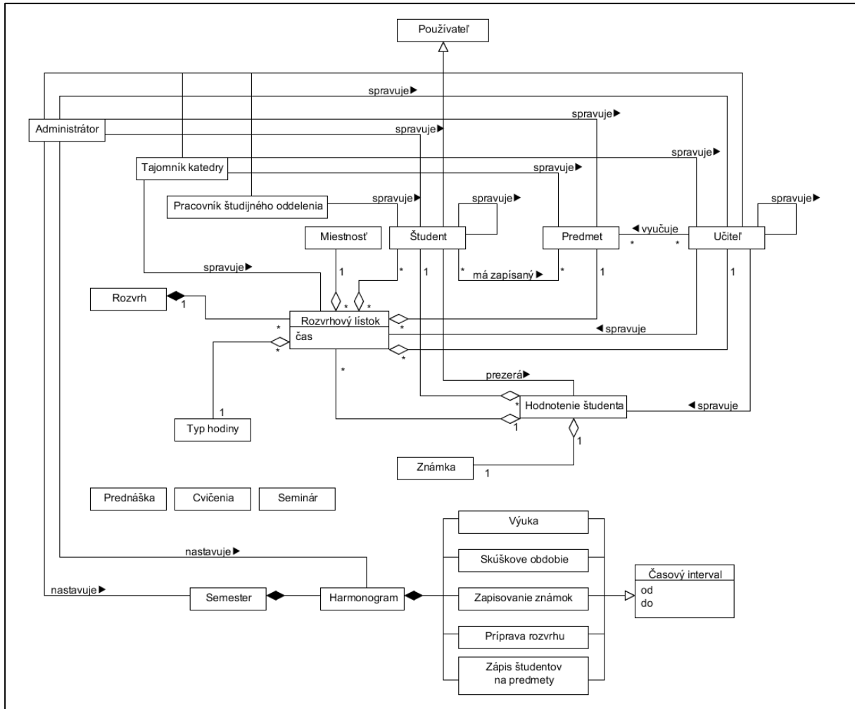
Obrázok 1: Doménový diagram
