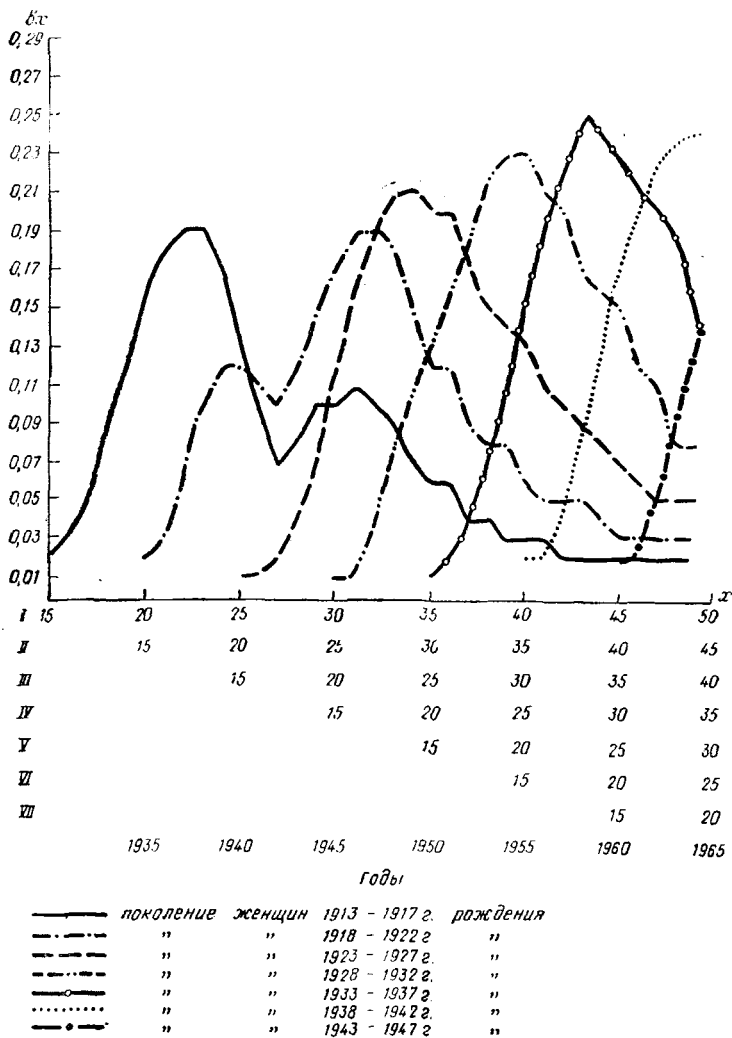
Рис. 1. Повозрастные вероятности вступления в первый брак для женщин СССР по поколениям
