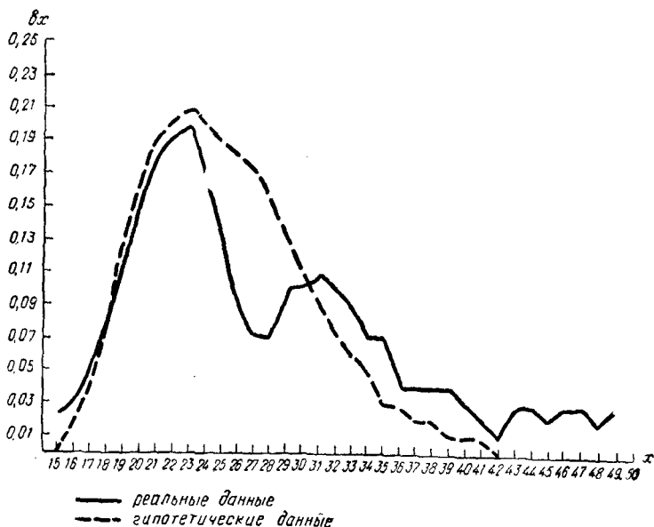
Рис. 2. Повозрастные вероятности вступления в первый брак для женщин РСФСР 1913—1917 гг. рождения
