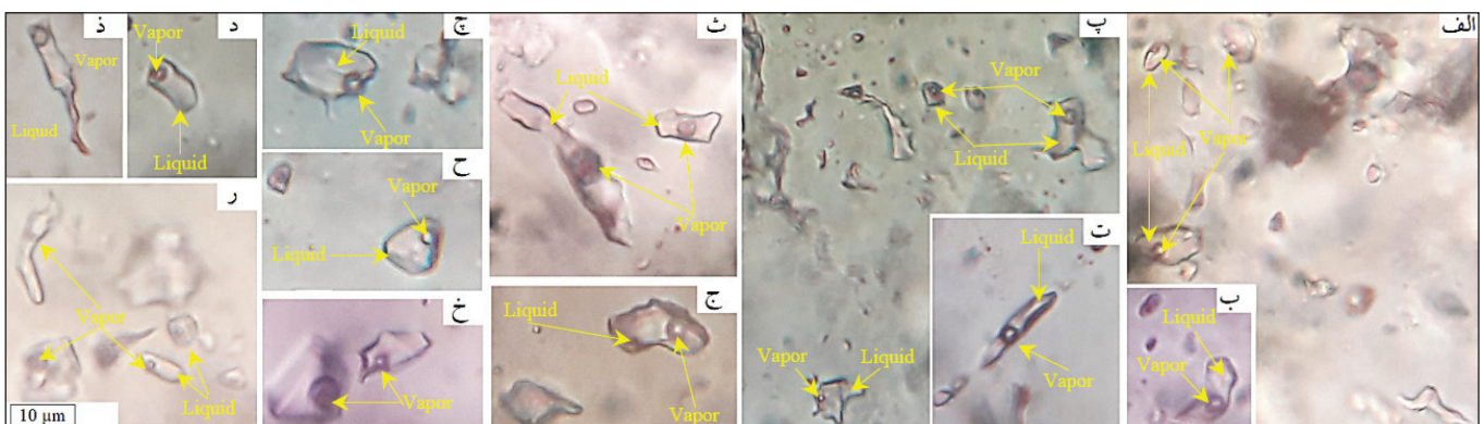
شکل ۸- الف و ب) میانبرهای سیال کانی کوارتز در رخساره تغذیه کننده؛ پ و ت) میانبرهای سیال کانی باریت در رخساره تغذیه کننده؛ ث) میانبرهای سیال کانی کوارتز در رخساره توده‌ای؛ ج و ح) میانبرهای سیال کانی اسفالریت در رخساره توده‌ای؛ ح و خ) میانبرهای سیال کانی باریت در رخساره توده‌ای؛ د، ذ و ر) میانبرهای سیال کانی باریت در رخساره لایه‌ای.
