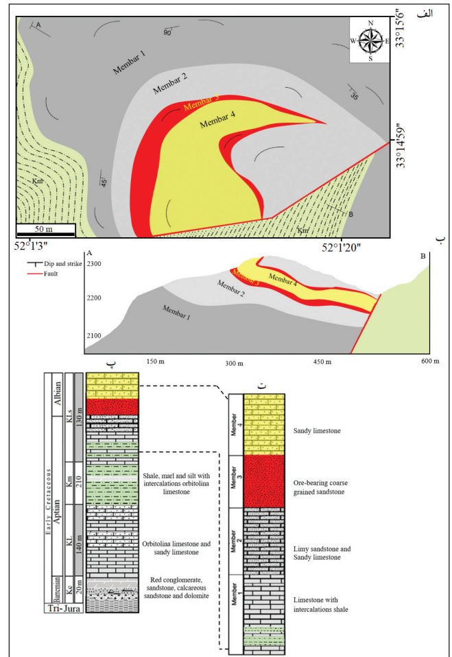
شکل ۲- الف) نقشه زمین‌شناسی کانسار یزدان؛ ب) مقطع زمین‌شناسی شمال باختری-جنوب خاوری کانسار یزدان؛ پ) ستون چینه‌شناسی عمومی کرتاسه زیرین در منطقه مورد مطالعه؛ ت) ستون چینه‌شناسی کانسار یزدان (واحدهای سنگی نقشه و مقطع زمین‌شناسی با عنوان عضو یک تا چهار معرفی شده‌اند که در ستون چینه‌شناسی (شکل ت) هر یک توصیف گردیده است).
