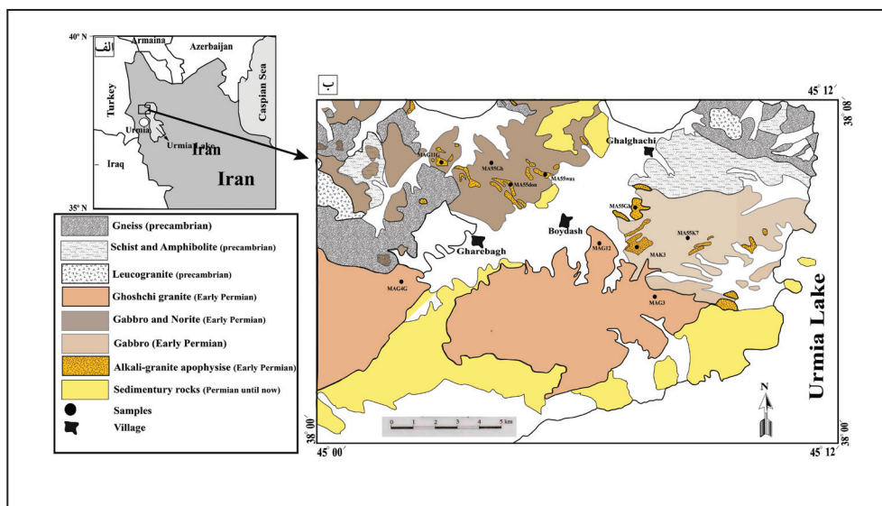
شکل ۱- نقشه زمین‌شناسی ساده شده از منطقه قوشچی، در باختر دریاچه ارومیه (برگرفته از خداینده و امینی فضل، ۱۳۷۲)، همراه با نقاط نمونه‌برداری.
