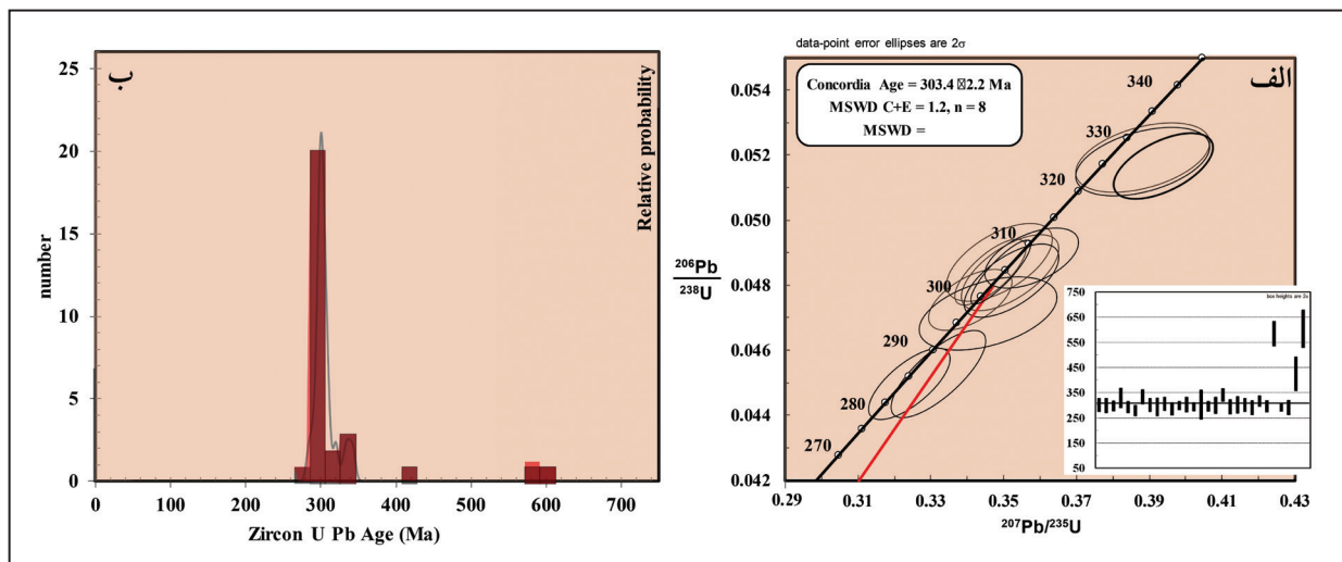
شکل ۷- الف) نمودار Concordia، U-Pb و ب) نمودار هیستوگرام با میانگین وزنی داده‌های سن‌سنجی زیرکن‌های پیکره‌های کوچک اسیدی قوشچی.
