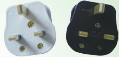
Y238 13A Plug (UF) (KM570473)
