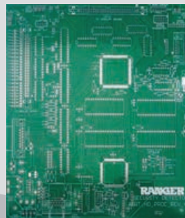
2 Layers PCB (#HD-PROC)
