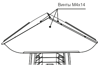
Рис. 7 – Установка козырька
