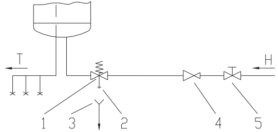
Схема підключення водонагрівача до водопровідної системи
