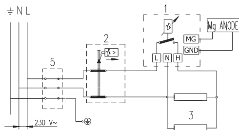
Электросхема
