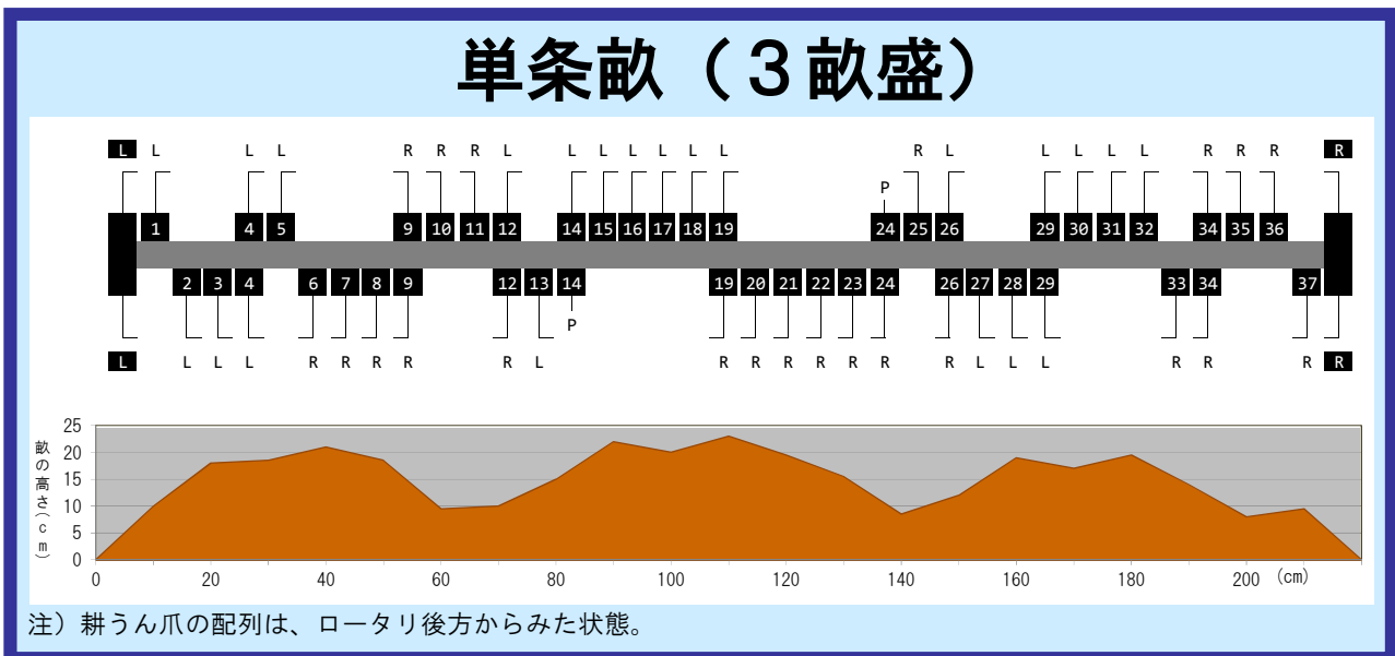
図31. アップカットロータリ (型式: BUR2210H) の耕うん爪配列と成形される畝の形状
