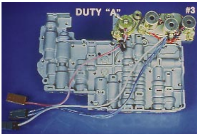
Shift Solenoid 3
