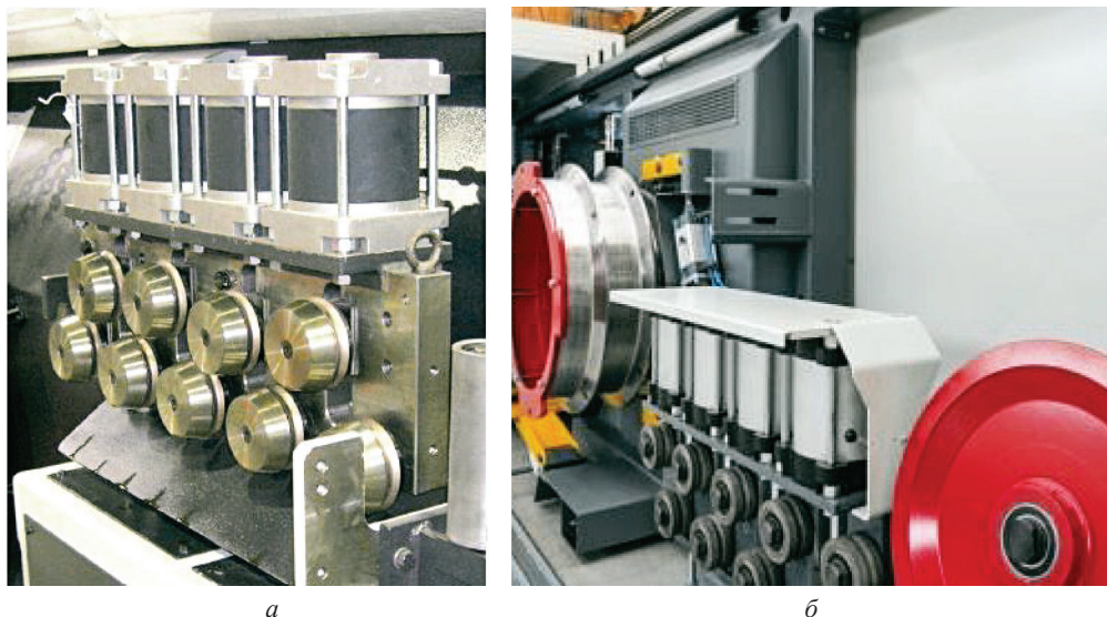
Рис. 3. Рихтовальное устройство станов холодной прокатки фирмы «Promostar S.r.l.» (а) 1 ; «Eurolls S.p.A.» (б) 2
